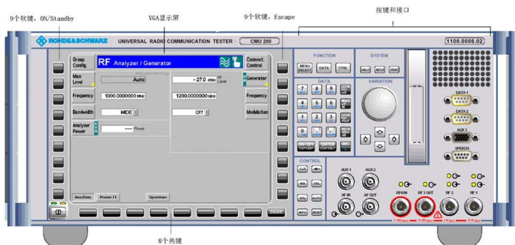
图 2-1 CMU200 前视图
