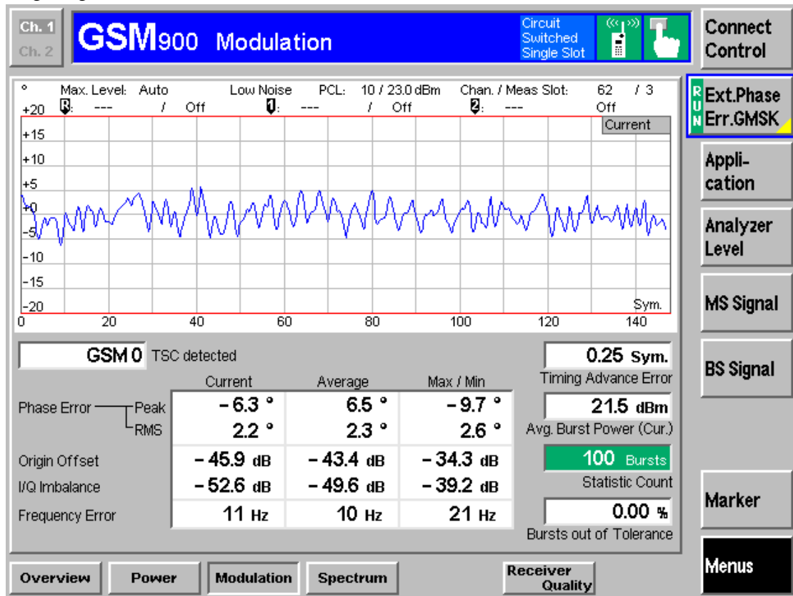
图 2—34 GSM900 Modulation
