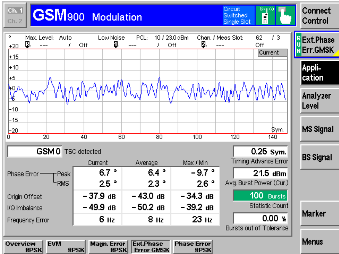
图 2—36 GSM900 Modulation_Application
