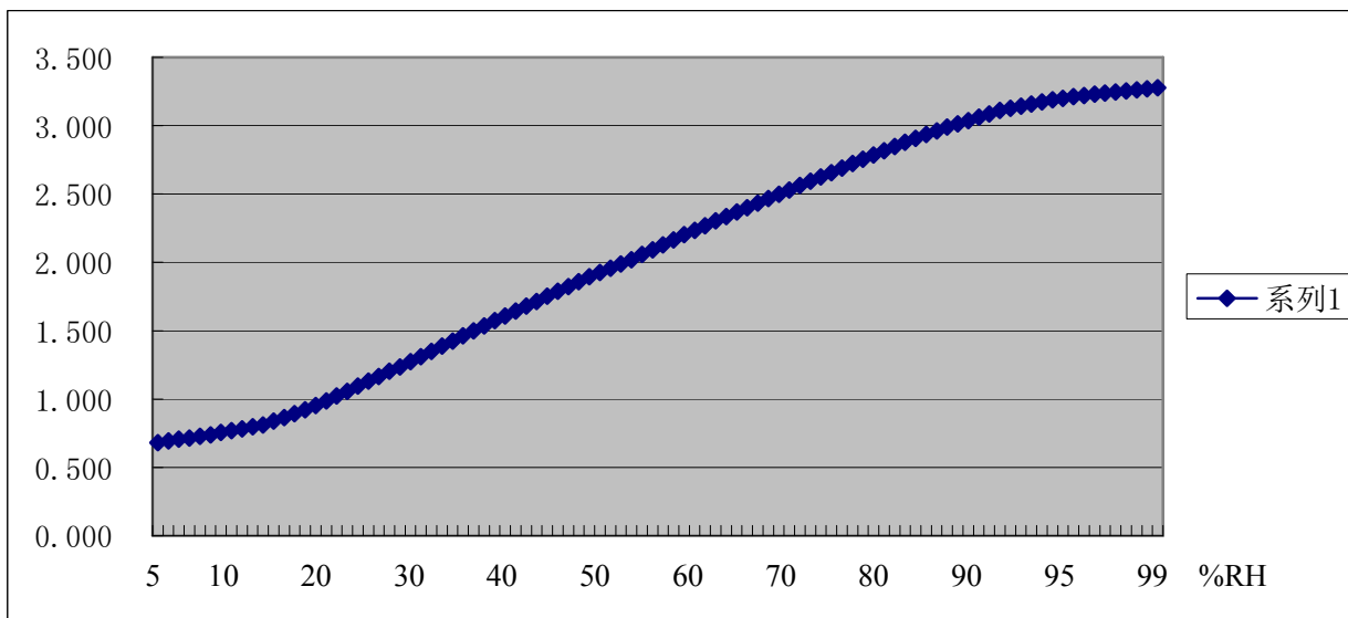
湿度输出电压特性
