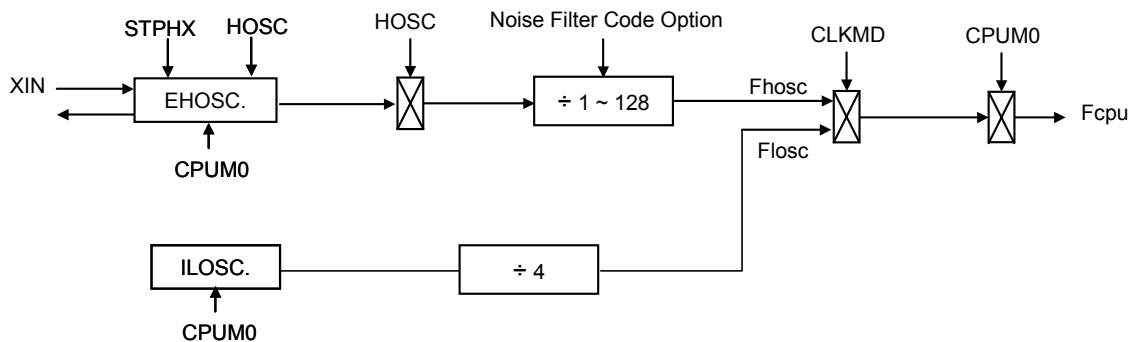
图 4-1 时钟框图
