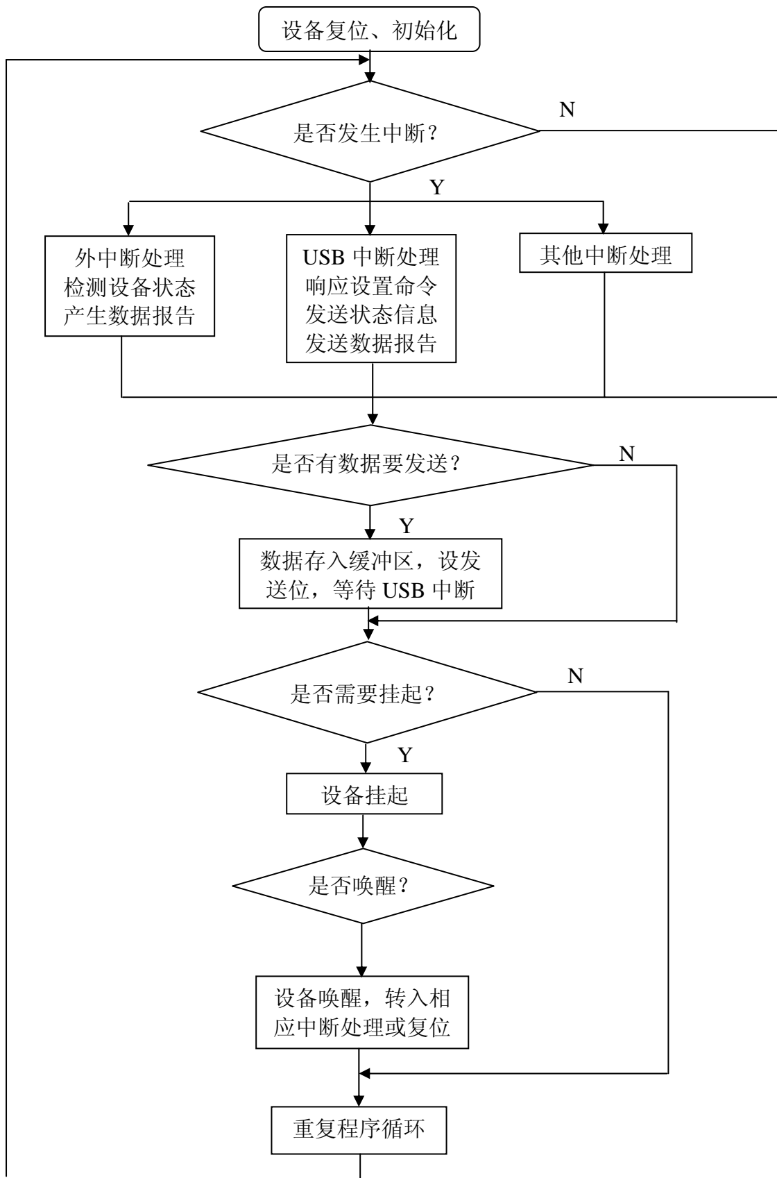
USB 协议栈固件流程图
