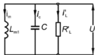
图 6 脉冲下降阶段的等效电路
