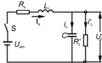
图 4 图 3 的简化电路
