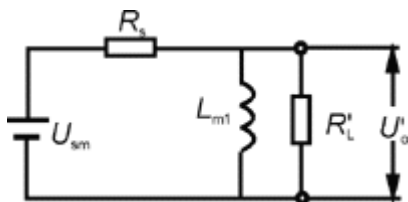
图 5 图 3 的低频等效电路
