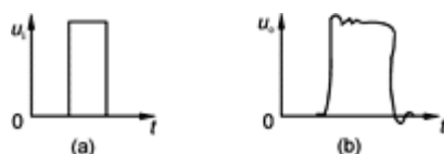
图 1 脉冲变压器输入、输出波形
