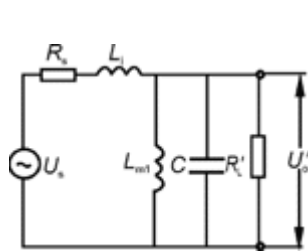
图 3 图 2 的等效电路
