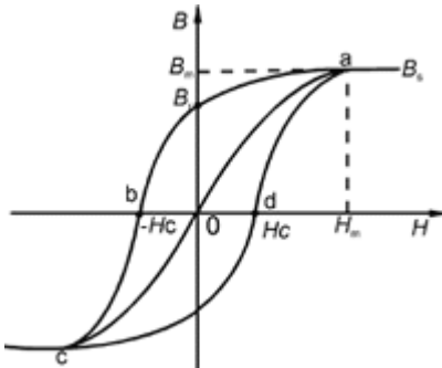
图 7 不带气隙的磁滞回线
