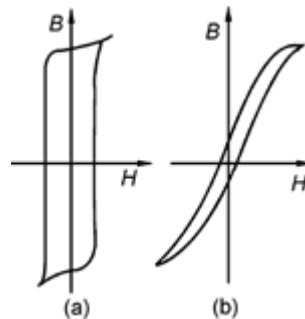
图 8 硬/软磁性材料和磁滞回线
