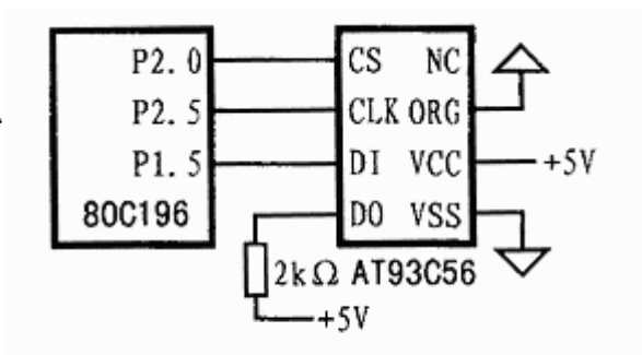
图2 AT93C56同80C196的硬件连接
