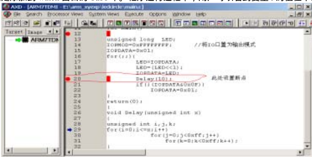
图 8.13 设置断点
