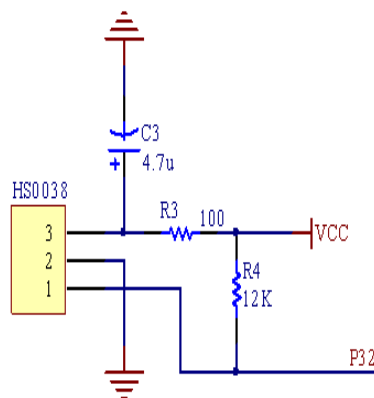
图 3 红外接收电路
