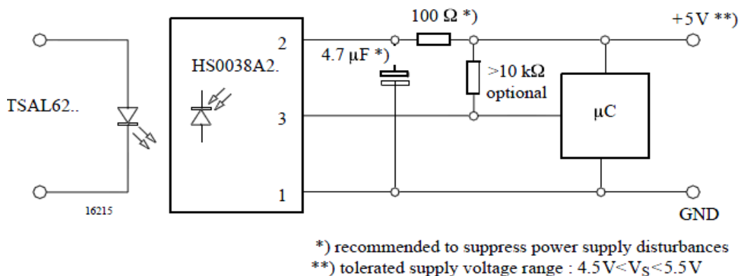
图 6 HS0038 的应用电路
