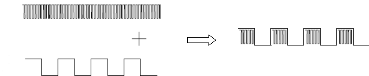
图 4 二进制码的调制
