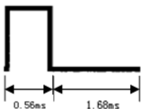
图 7 二进制码'1'
