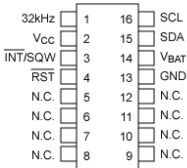
图 1. DS3231 引脚配置
