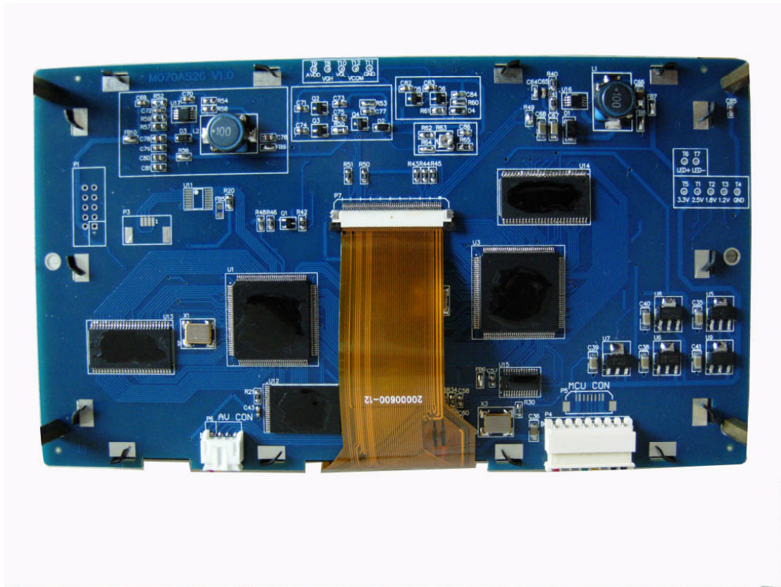
图 2 实物照片（背板）
