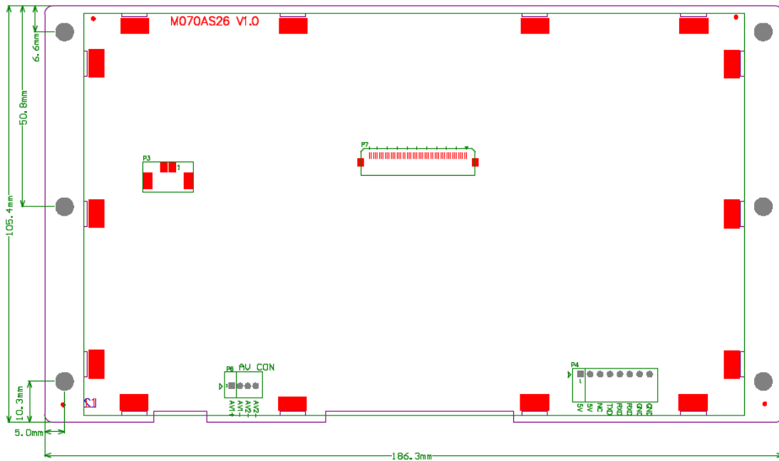
图 1 模块外形尺寸
