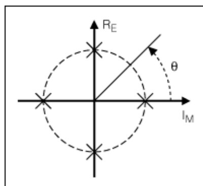
QPSK 调制示意图
